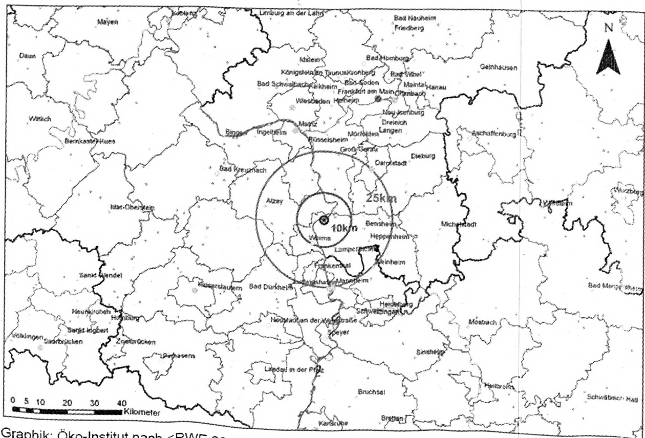
Abbildung 4.1: Katastrophenschutzzonen um das KKW Biblis
